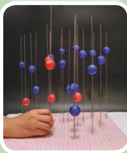
图3-4-4 搭建碳、氧原子
