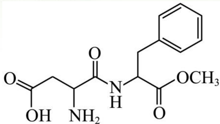
阿斯巴甜
