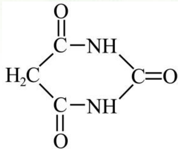
巴比妥酸
